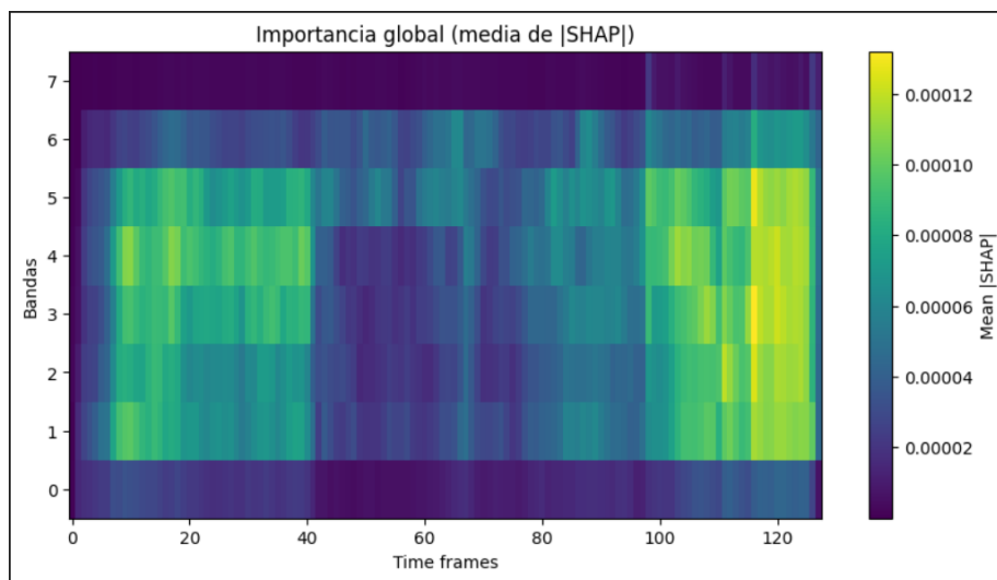
Figura 33: Shap general de los espectrogramas
