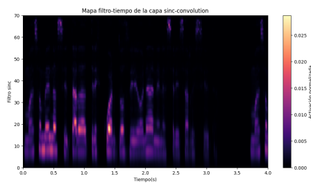
(a) Mapa filtro-tiempo de la capa sinc-convolution.
