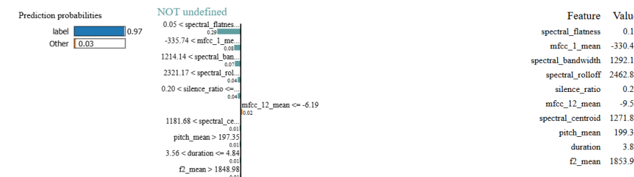
Figura 47: Explicación local con LIME
