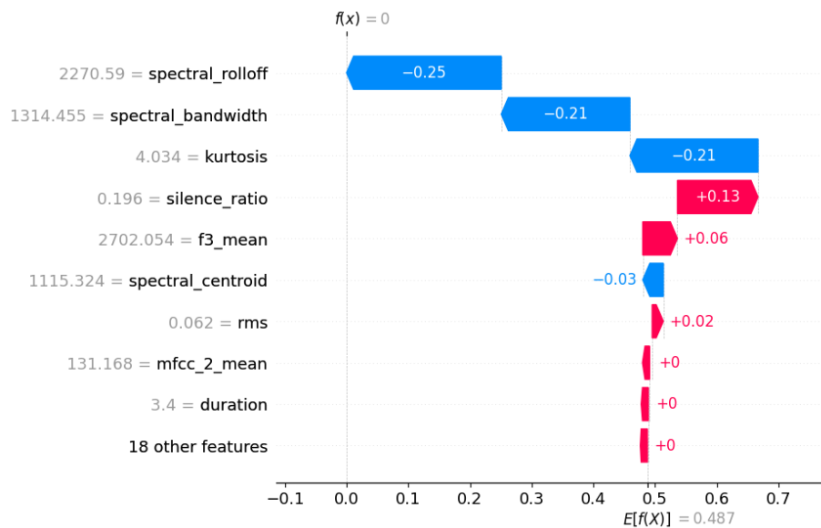
Figura 53: Explicación local con SHAP tras quitar spectral flatness y mfcc 1
