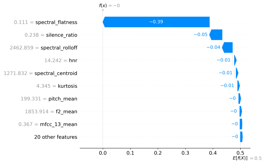
Figura 41: Explicación local con SHAP
