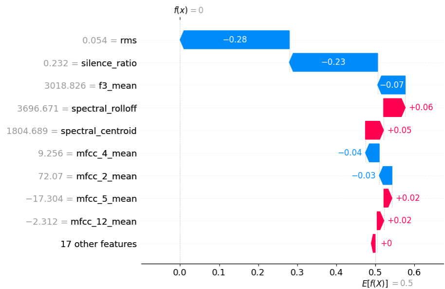
Figura 46: Explicación local con SHAP tras quitar spectral flatness, mfcc 1 y spectral bandwidth
