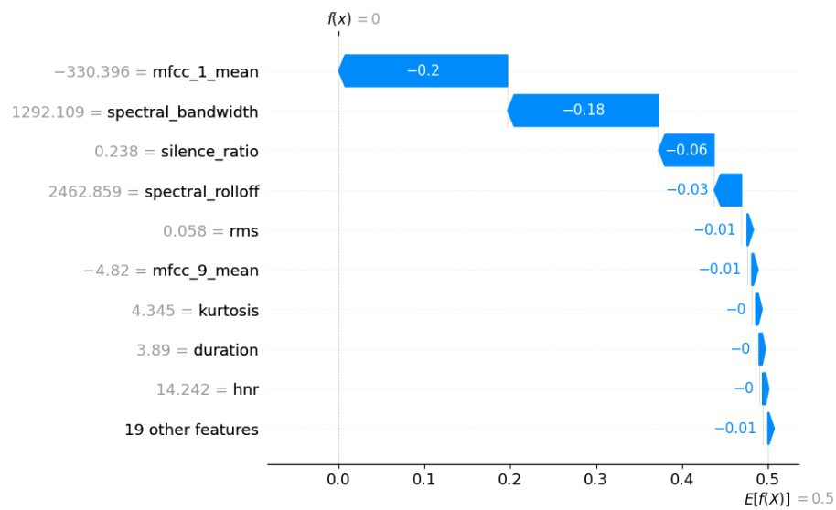
Figura 43: Explicación local con SHAP tras quitar spectral flatness
