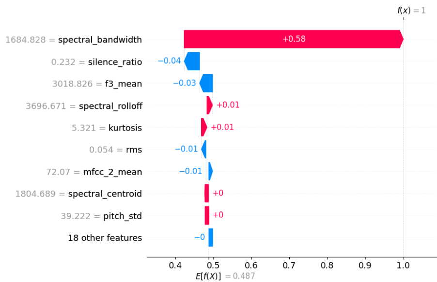
Figura 52: Explicación local con SHAP tras quitar spectral flatness y mfcc 1
