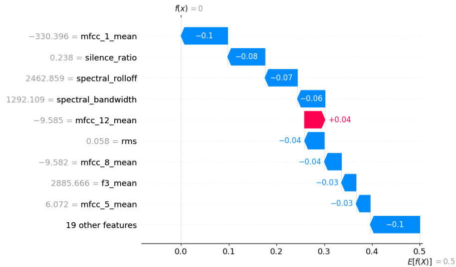
Figura 57: Explicación local con SHAP tras quitar spectral flatness
