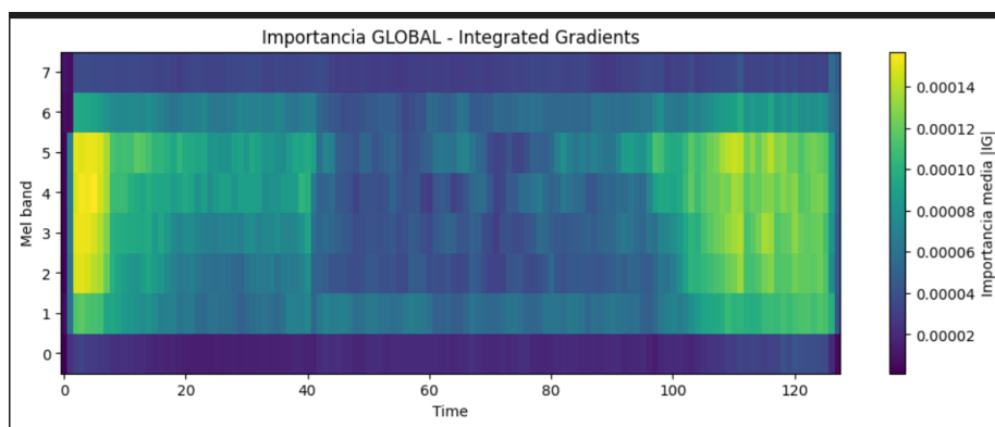
Figura 37: Integrated gradients general de los espectrogramas
