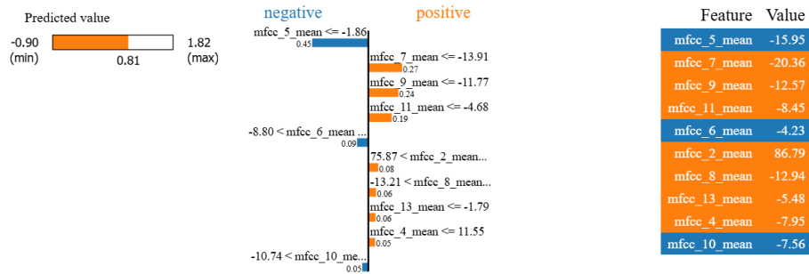
Figura 28: Influencia general de las características.
