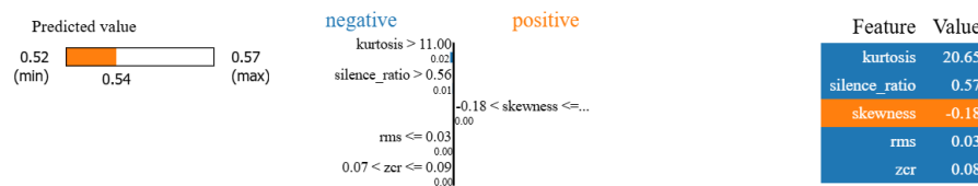
Figura 24: Influencia general de las características.
