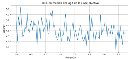
(a) Resultados de “logit” usando RISE.
