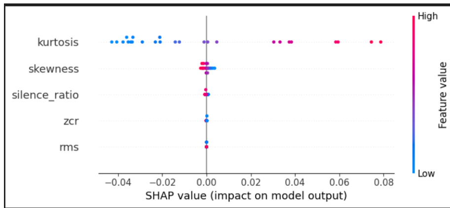
Figura 14: Influencia general de las características.
