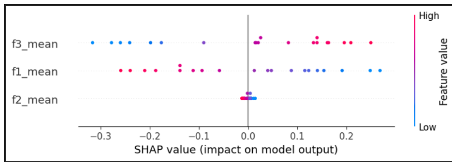
Figura 20: Influencia general de las características.
