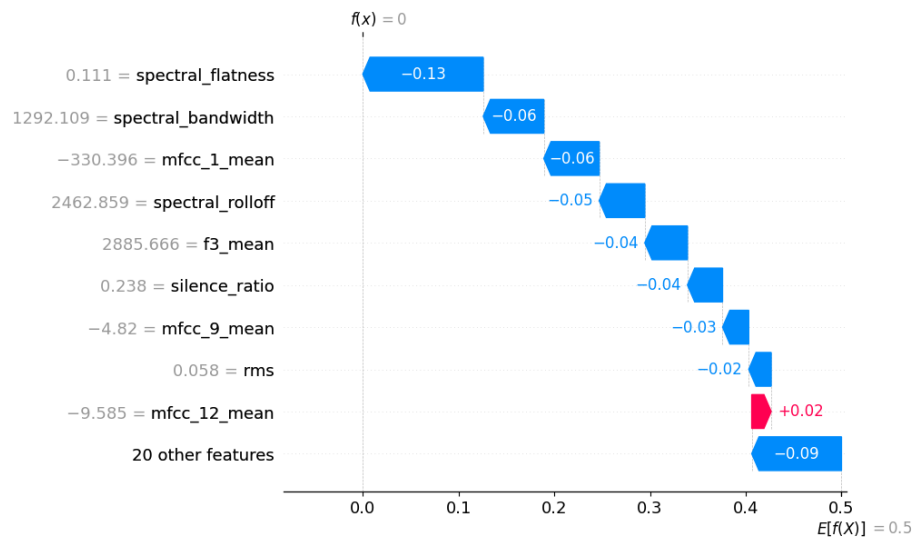
Figura 54: Explicación local con SHAP
