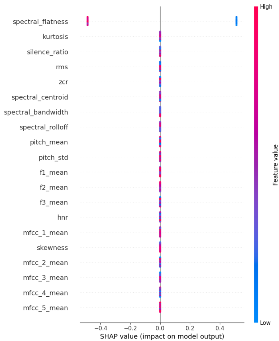
Figura 49: Explicación global con SHAP
