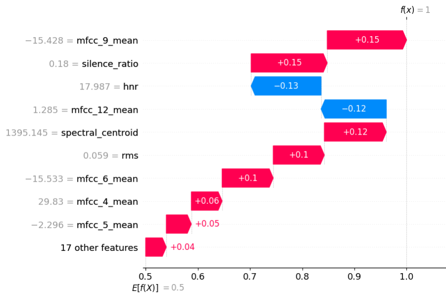
Figura 59: Explicación local con SHAP tras quitar spectral flatness, mfcc 1 y spectral bandwidth
