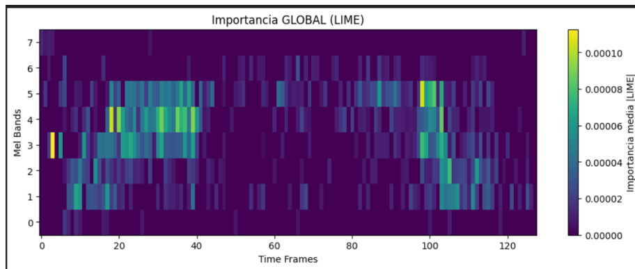
Figura 35: Lime general de los espectrogramas
