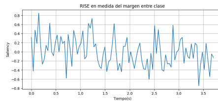
(b) Resultados de “margin” usando RISE.
