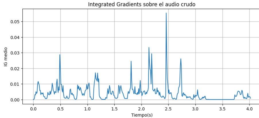
Figura 11: Importancia temporal según IG sobre audio.
