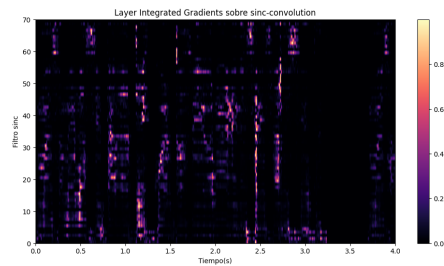
(b) Mapa filtro-tiempo normalizado generado por IG.
