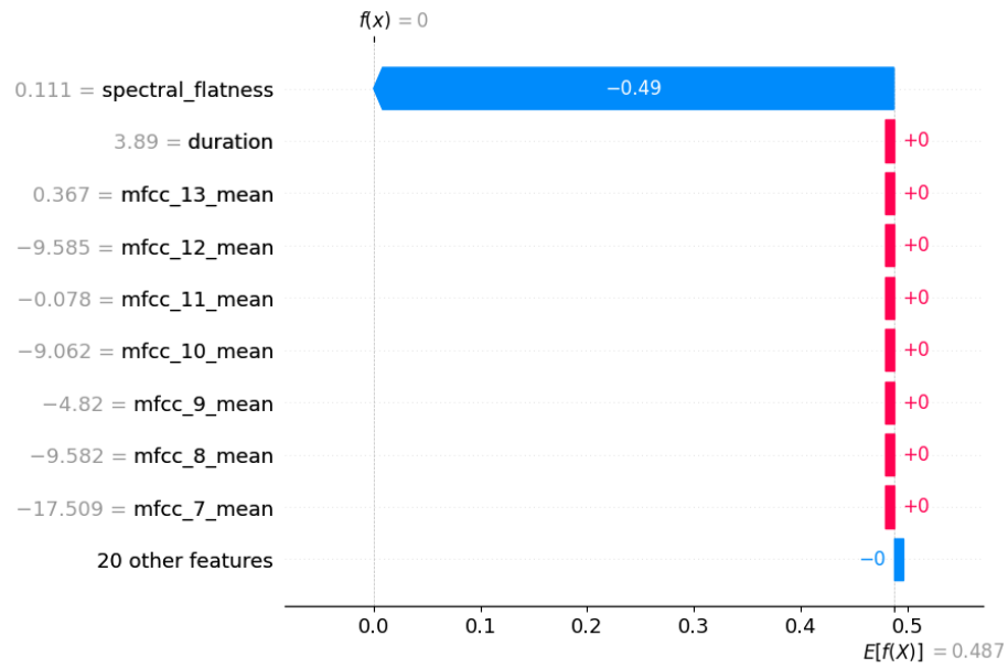
Figura 48: Explicación local con SHAP
