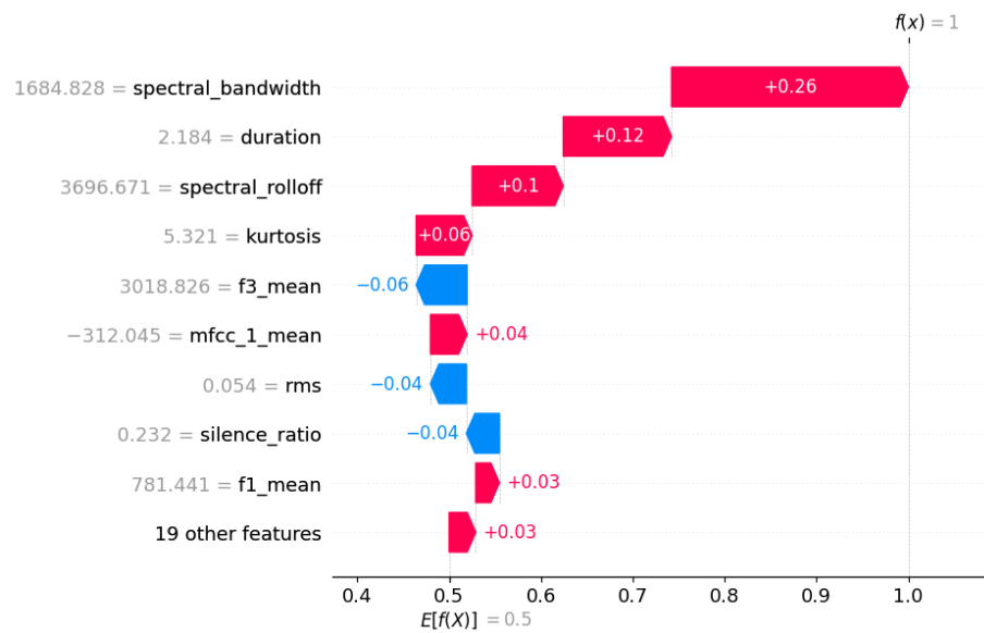
Figura 44: Explicación local con SHAP tras quitar spectral flatness
