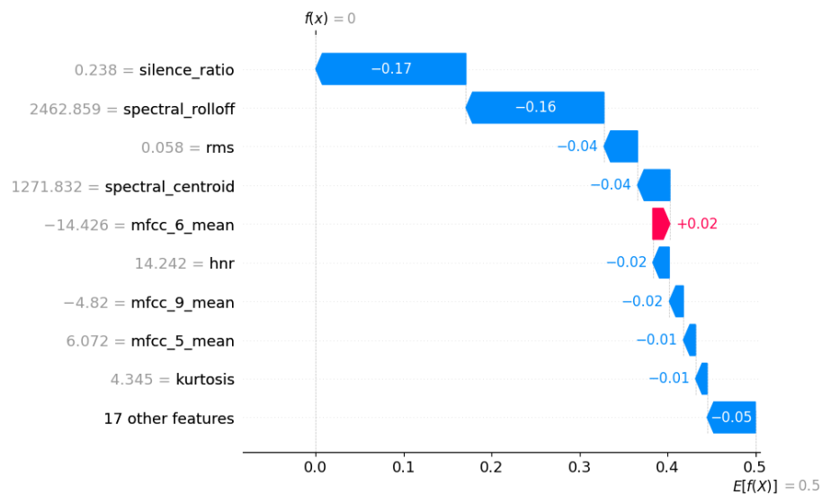
Figura 45: Explicación local con SHAP tras quitar spectral flatness, mfcc 1 y spectral bandwidth
