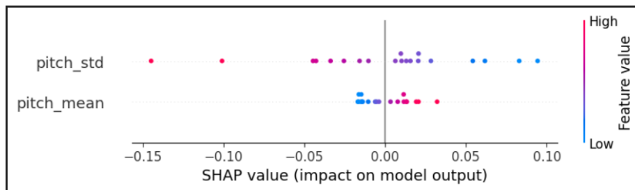
Figura 18: Influencia general de las características.
