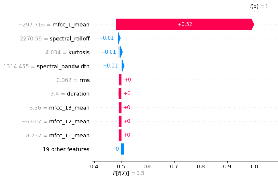
Figura 51: Explicación local con SHAP tras quitar spectral flatness
